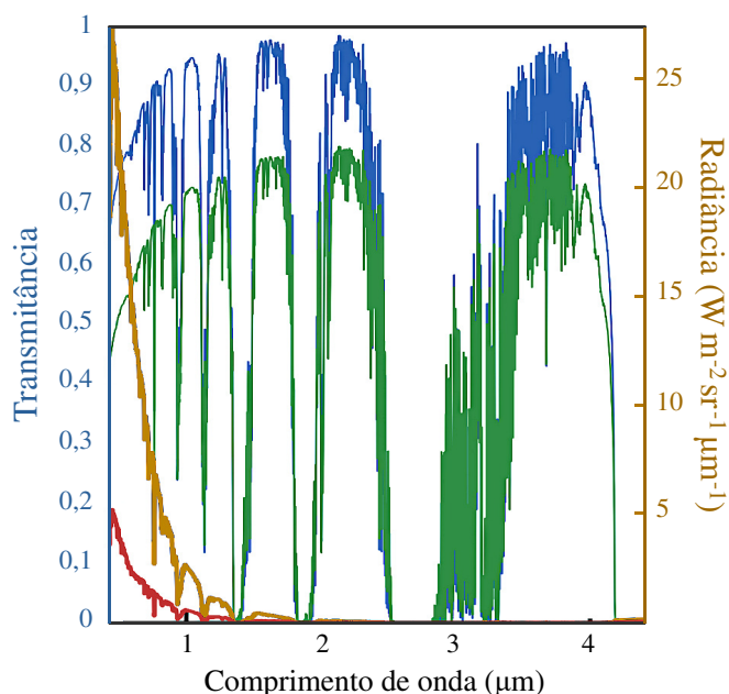
Fig. 1. Transmitância e radiação espectral em função do comprimento de onda, nas cidades de Tucson, Arizona (azul e ouro, respectivamente), seca, no verão, e Waterford, Irlanda (verde e vermelho), úmida, encoberta [17].
