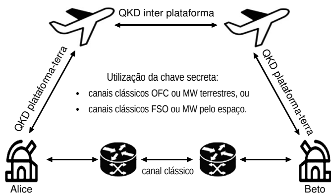
Fig. 3. QKD via HAP, MAP ou LAP. Uma vez que a chave é distribuída de forma segura, a comunicação cifrada pode ocorrer por canais clássicos terrestres ou aeroespaciais (figura baseada em [41]).
